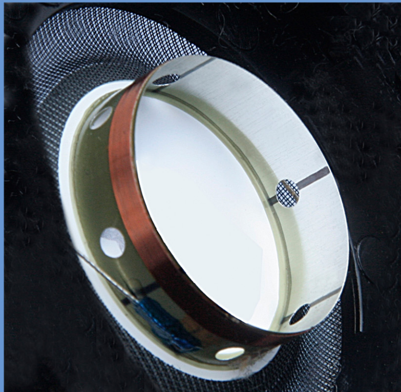
Super precisie aluminium spreekspoel met koelsleuven
