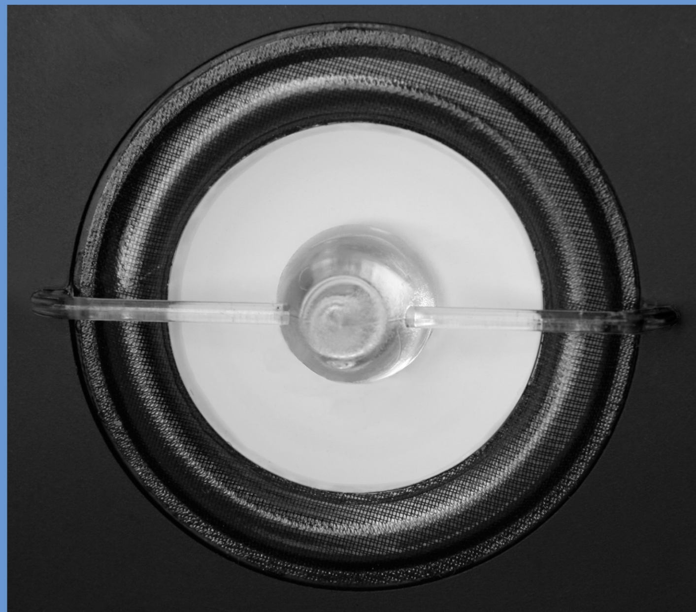
Keramische inverted dome met faseplug voor coherente afstraling
